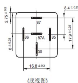
底视图 Bottom View
