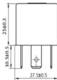
外形图 External Dimentions
